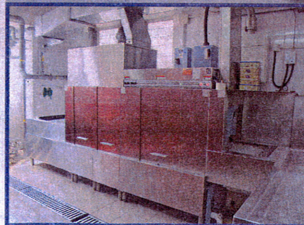
■ 卓滙特別為大榮華工場設計的長龍式洗碗碟機，無論長度、清洗及烘乾功能，都是按照客人的需要而度身訂造的。
