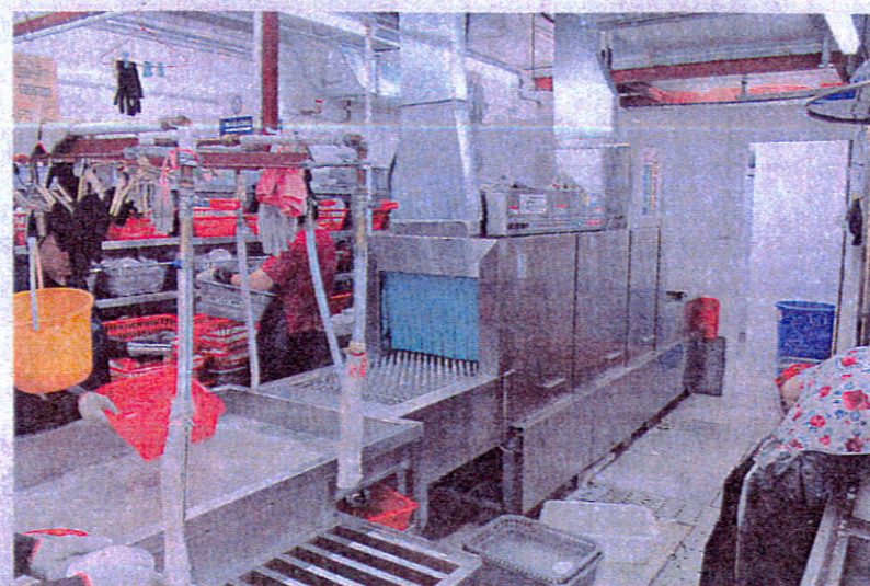
■ 卓滙特別為大榮華工場設計的長龍式洗碗碟機，無論長度、清洗及烘乾功能，都是按照客人的需要而度身訂造的。
